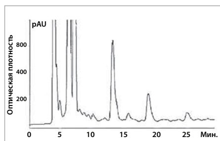
Рис. 3. Хроматограмма антимикробных метаболитов штамма закваски Биотроф-600
