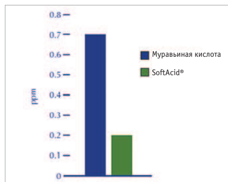
Рис. 2. Скорость испарения муравьиной кислоты (результаты получены в Felleskjøpet, Норвегия), ppm — частей на миллион
