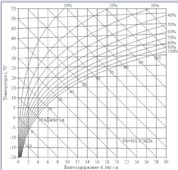
Рис. 1. I-d-диаграмма влажного воздуха
